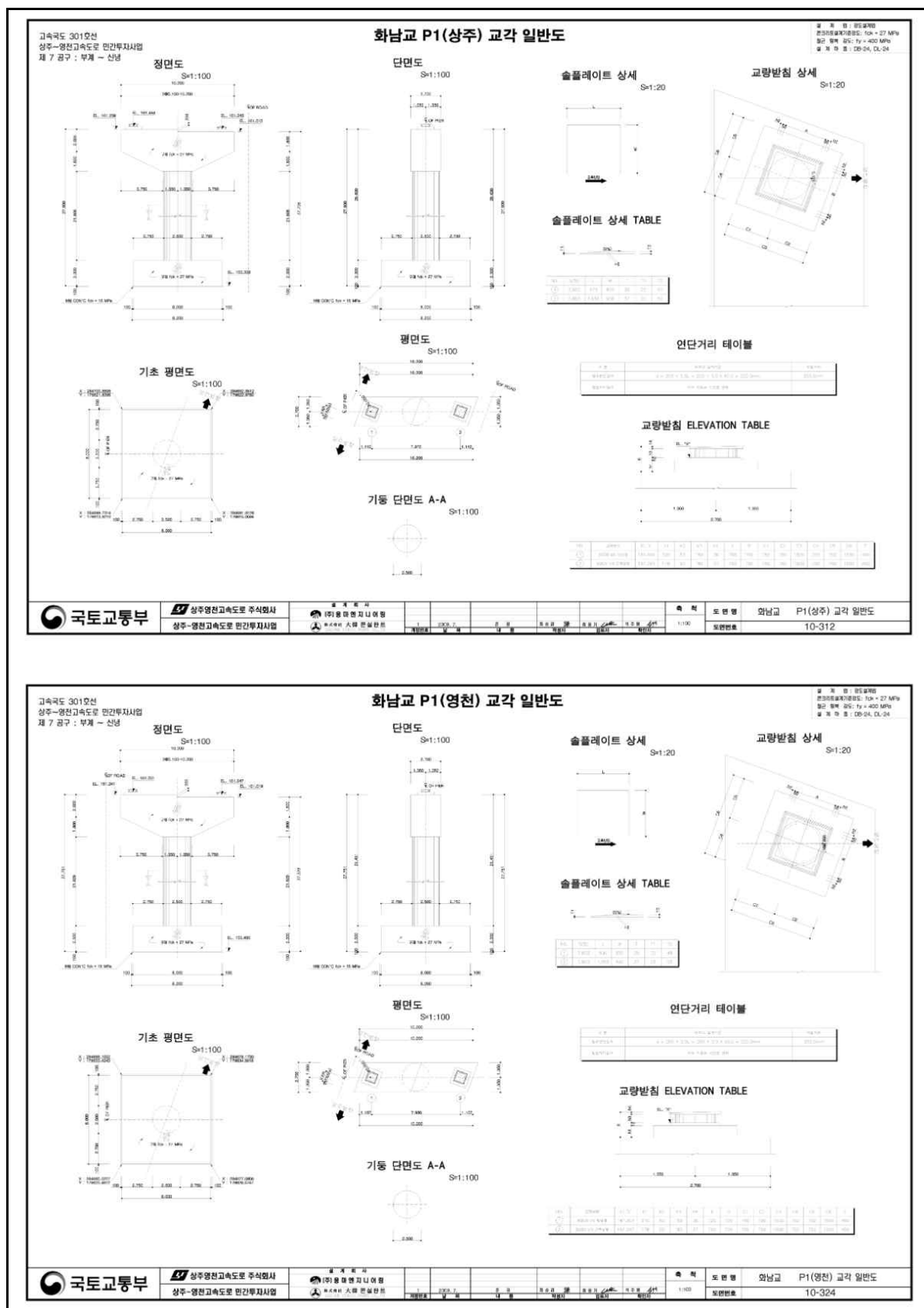
【그림 23.1.7】 교각 일반도
