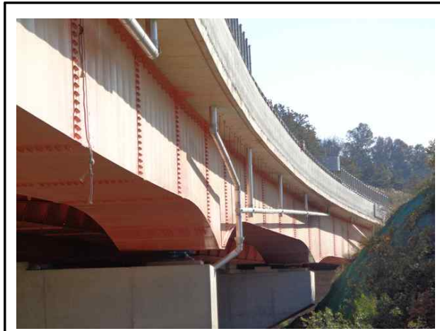
배수관 전경
