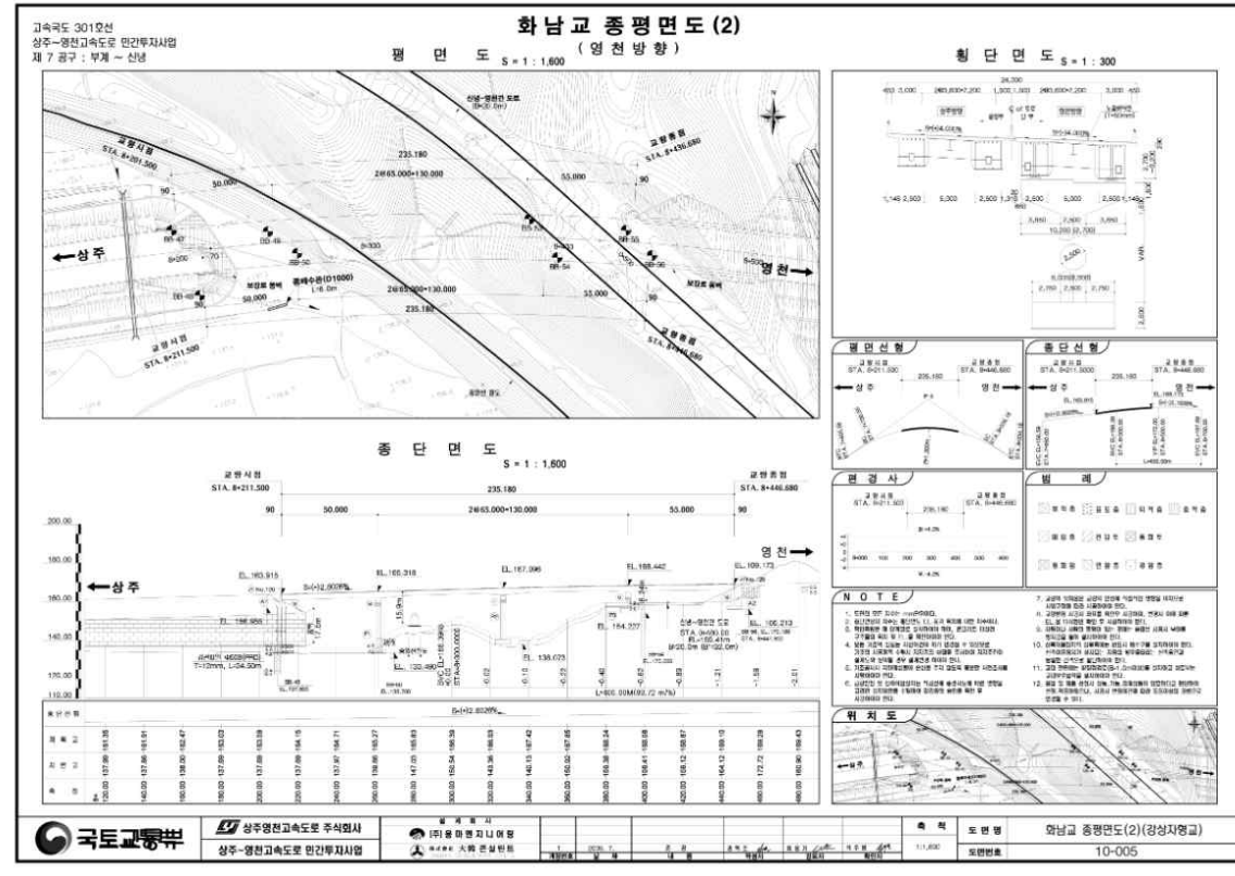
【그림 23.1.3】 종평면도
