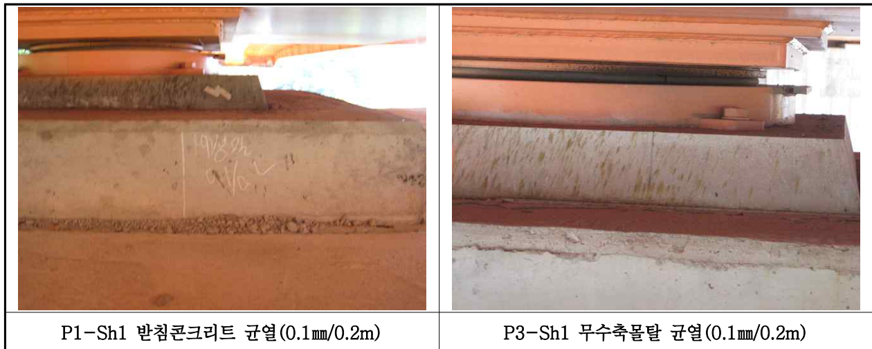
【사진 23.3.36】 교량받침 손상현황
